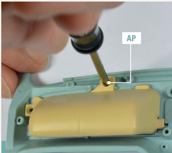
74-7. Ziehen Sie eine Schraube AP im oberen Loch des Schalttafelkastens fest, um ihn zu fixieren.
