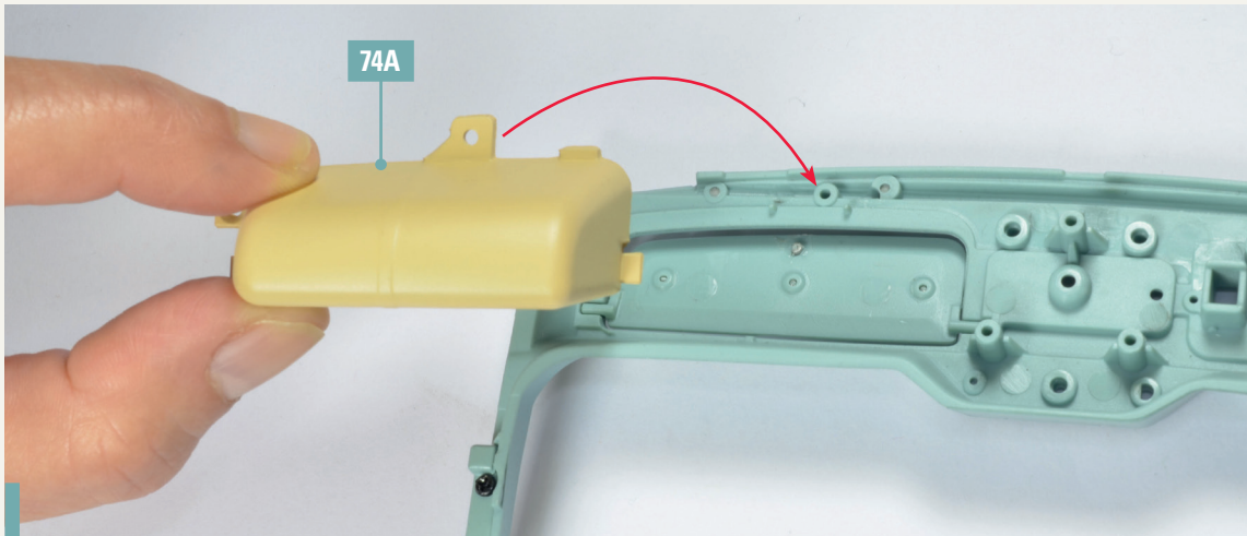
74-5. Setzen Sie den Schalttafelkasten 74A auf die Baugruppe.
