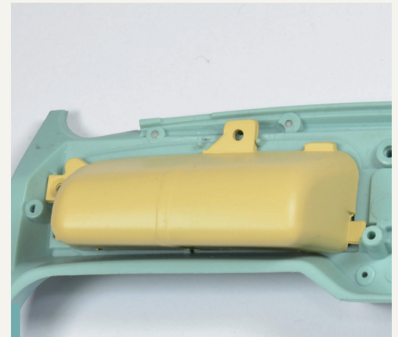
74-6. Vergleichen Sie anhand des Fotos, ob der Schalttafelkasten korrekt positioniert ist.
