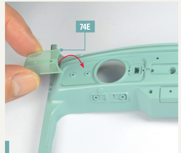
74-9. Setzen Sie auf der Außenseite des Armaturenbretts das große Ziergitter 74E wie gezeigt ein.
