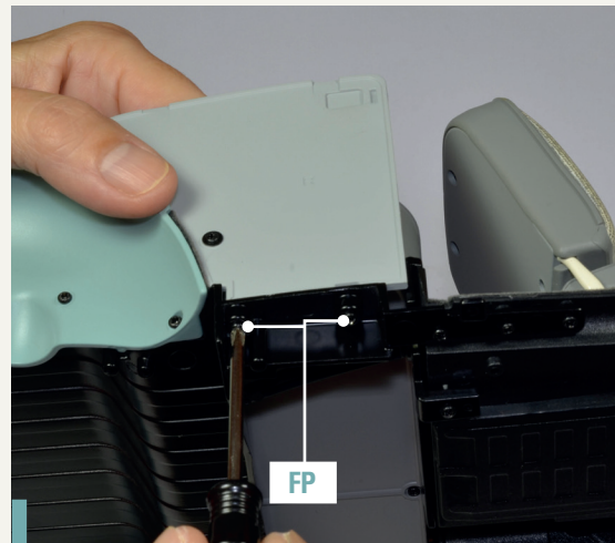
50-8. Befestigen Sie die Blende mit zwei Schrauben FP am Kofferboden.
