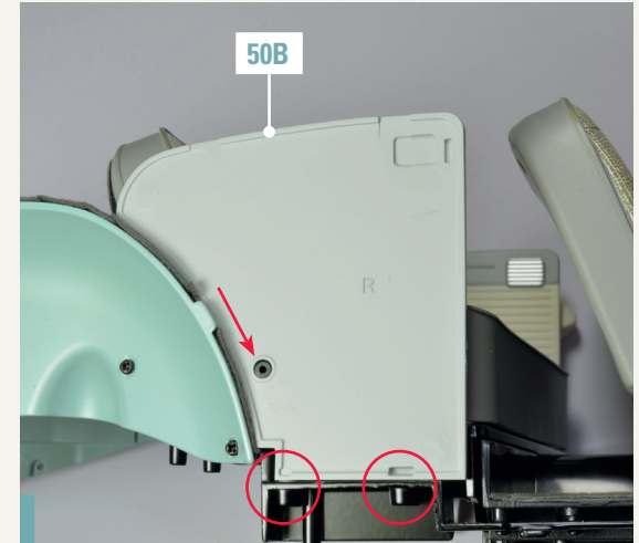
50-6. Bauen Sie die rechte hintere Innenverkleidung 50B am anderen Ende des Rücksitzes ein. Stecken Sie die beiden Stifte der Verkleidung in die entsprechenden Aussparungen am Kofferboden (siehe Kreise auf dem Foto) und die Lochsäule rechts von der Rückenlehne in das Loch in der Verkleidung (siehe Pfeil auf dem Foto).
