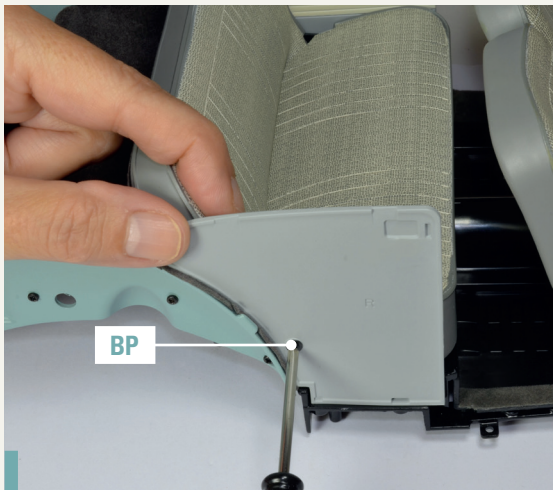
50-7. Befestigen Sie die Rückenlehne mit einer Schraube BP an der rechten Innenverkleidung. Ziehen Sie auch diese nicht vollständig fest.
